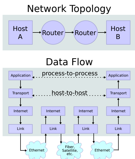
TCP/IP-gerelateerde protocollen
